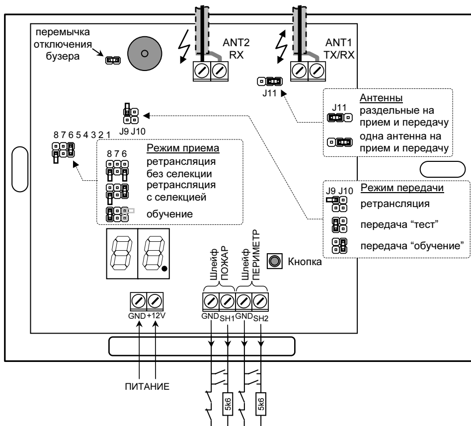
Рис. 3. Монтажная схема ретранслятора
