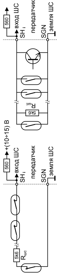
а) нормально замкнутые датчики
