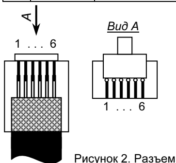
Рисунок 2. Разъем
